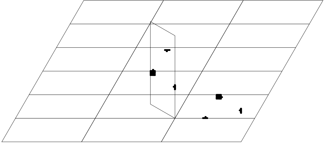
图 4: Non ergodic case
